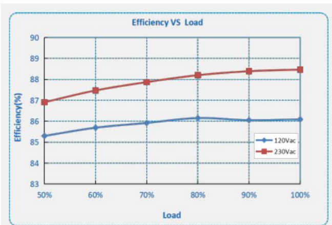
F1-060X-054 ( I_o=1.4A )
